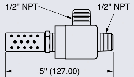
W00-10-918 QRV w/MUFFLER
