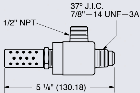
W00-10-917 QRV w/MUFFLER
